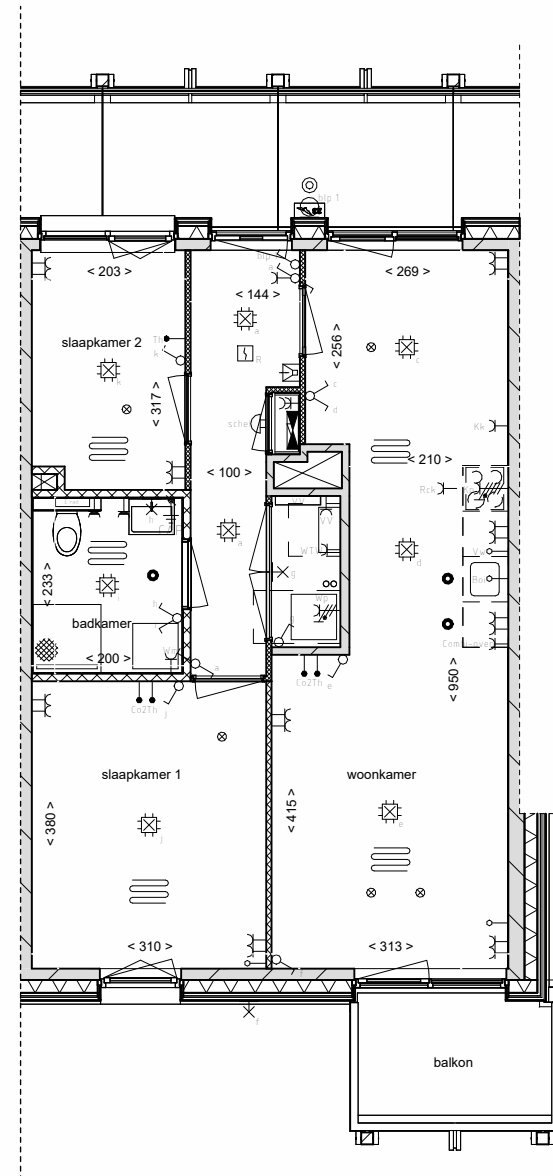
plattegrond
